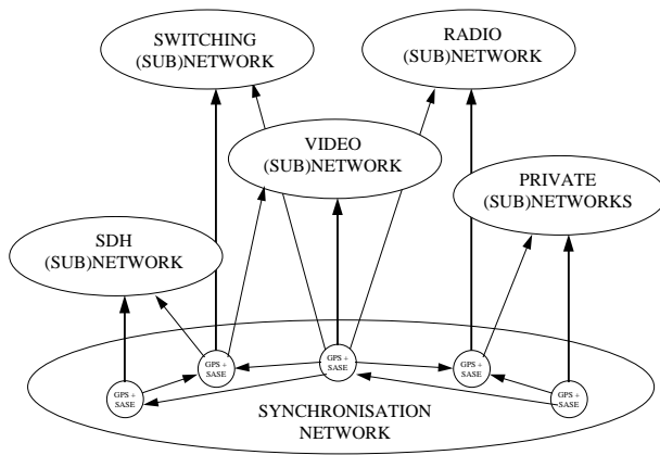
Figure 7 : Separate synchronisation network layer
